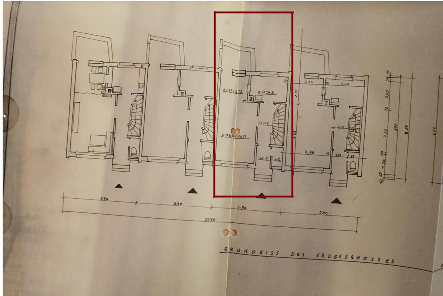
Grundriss Erdgeschoss
